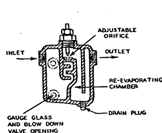
FIG. 29. FLASH TRAP
