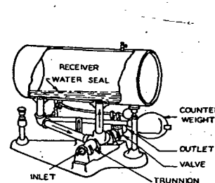
FIG. 31. TILTING TRAP
