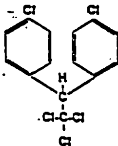
DDT
