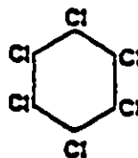
LINDANE
