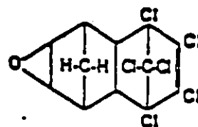
ENDRIN
