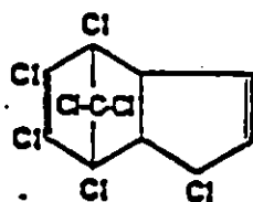
HEPTACHLOR
