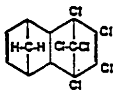
ALDRIN
