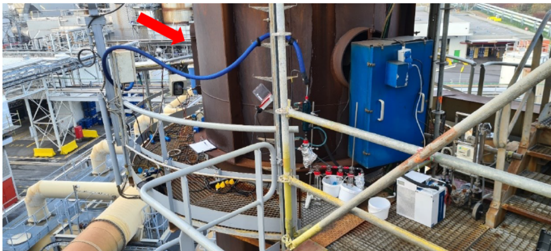
Figuur 1 : Meetpunt en gemodificeerde EPA OTM-45 opstelling schouwmeting op de DTO2 bij Indaver,
