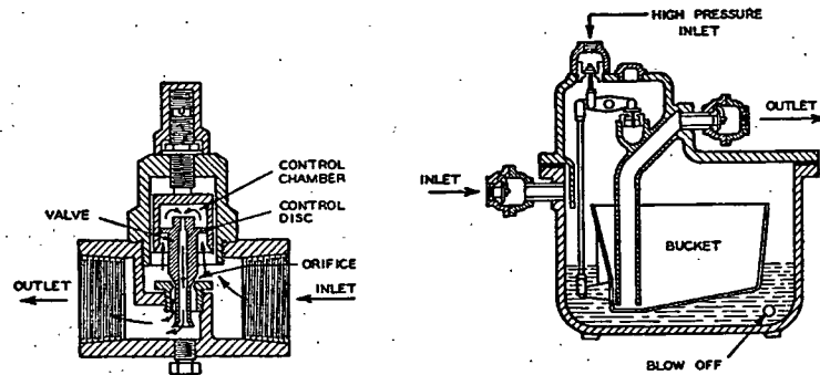
FIG. 33. IMPULSE TRAP
