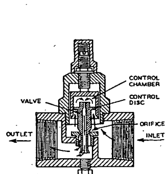
FIG. 33. IMPULSE TRAP
