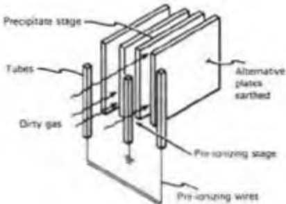
Tubular-Type Precipitator
