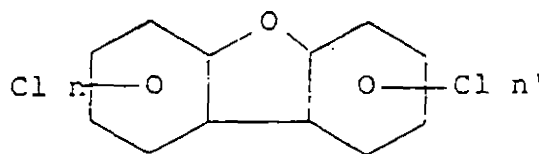
(n+n')-chlorodibenzofuran
