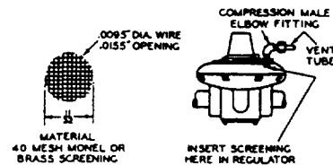
FIG. 11—Flame Check
