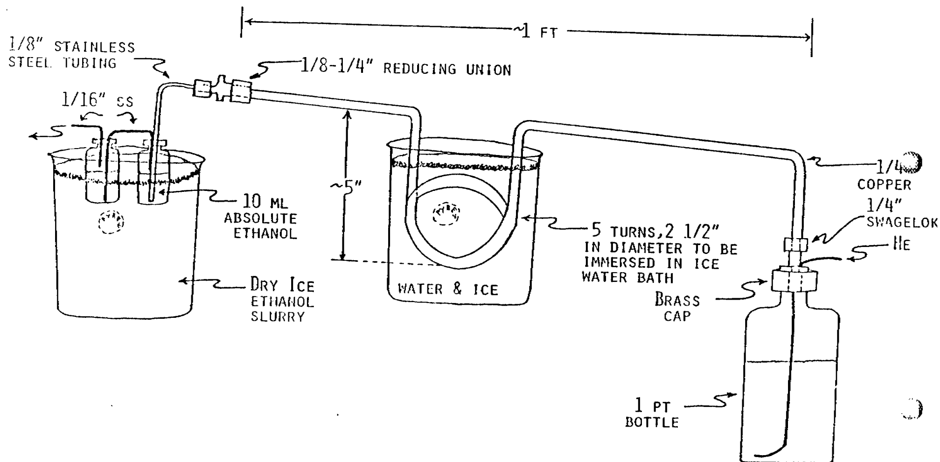
EFFLUENT TUBE DETAILS
