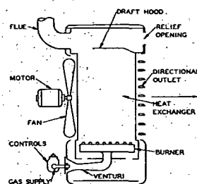
Fig. 12....Gas-Fired Propeller Fan Unit Heater
