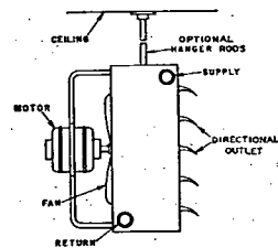
Fig. 6....Propeller Fan Unit Heater—Horizontal-Blow Type
