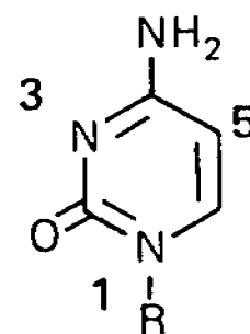
Cytosine
