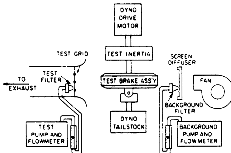
Fig. 1 - Dynamometer test schematic
