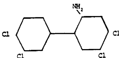
3',4,4',5-tetrachloro-2-biphenylamine
