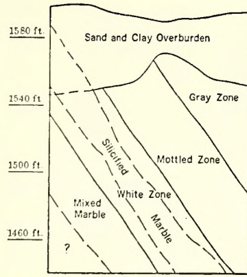
Section A-A' Scale: 1" = 80'
