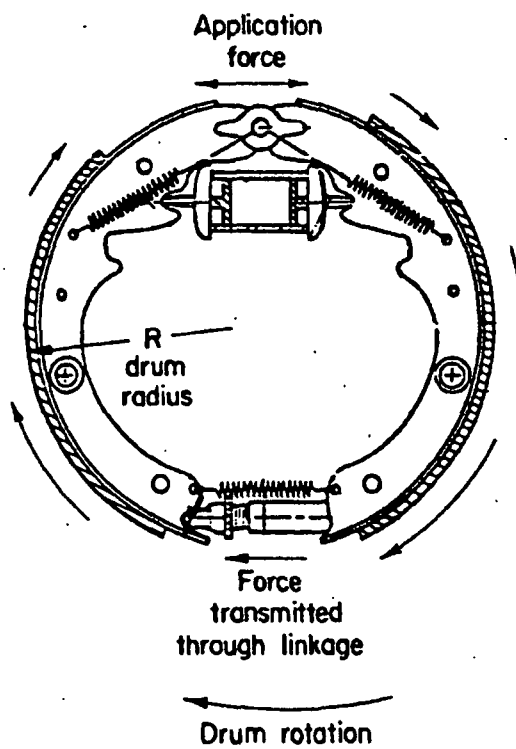
b. duo-servo
