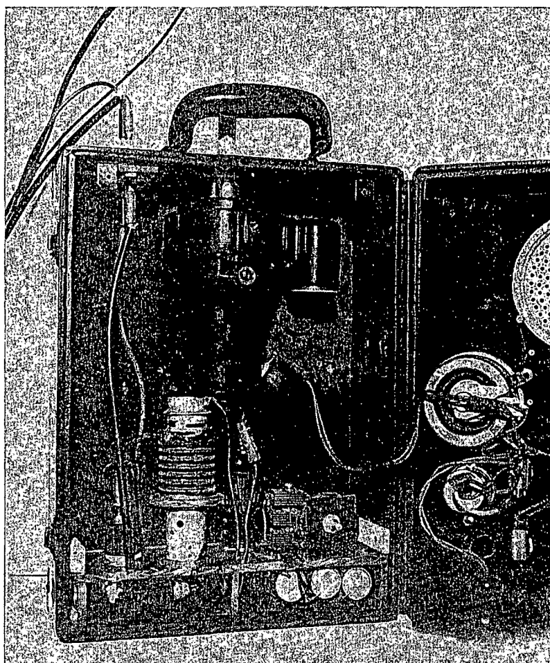
Fig. 2.—PHS-50 installed in the old M. S. A. case.
