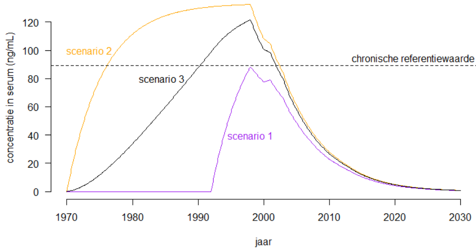
Figuur 2 Modelsimulatie van het lange termijn tijdverloop van de PFOA concentratie ( \text{ng mL}^{-1} ) in het serum van omwonenden in de binnenste contour over de periode 1970 – 2030 t.g.v. het inademen van PFOA.
