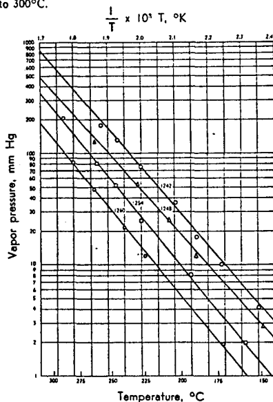
Fig. 3—VAPOR PRESSURES OF AROCLORS
