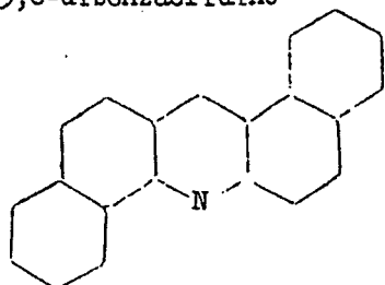
1,2,5,6-dibenzacridine
