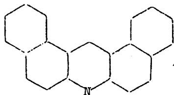
1,2,7,8-dibenzacridine
