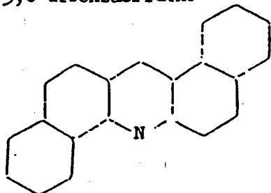
1,2,5,6-dibenzacridine
