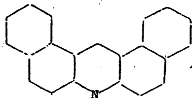
1,2,7,8-dibenzacridine
