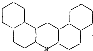
1,2,7,8-dibenzacridine
