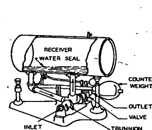
FIG. 31. TILTING TRAP
