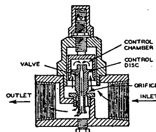
FIG. 30. IMPULSE TRAP
