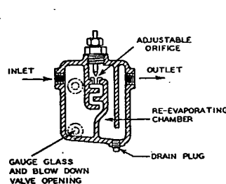
FIG. 29. FLASH TRAP
