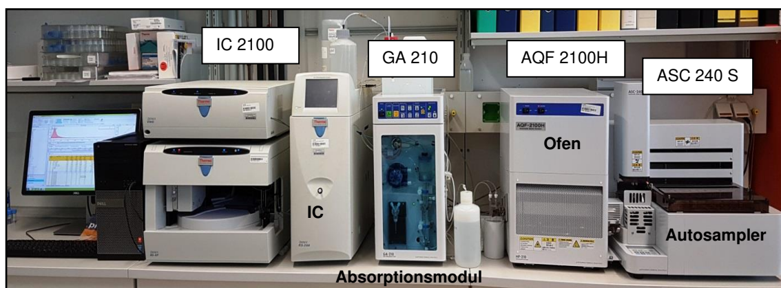
Abbildung 3-3. Verbrennungs-Ionen-Chromatographie-(CIC)-System
