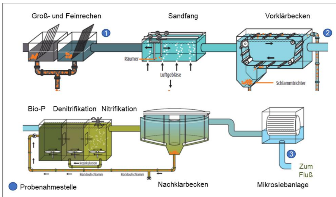
Abbildung 4-13. Schema der Kommunkläranlage der Entsorgungsbetriebe einer hessischen Großstadt (modifiziert nach ELW, 2010)
