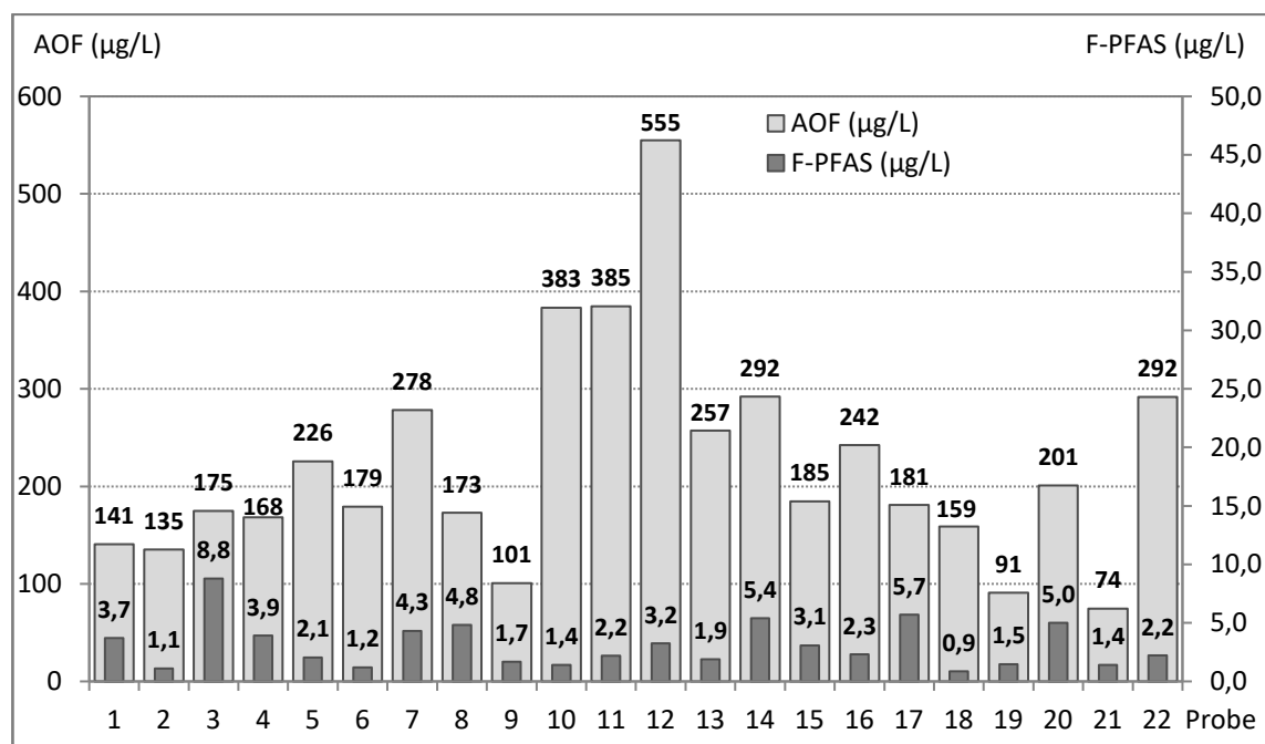
Abbildung 4-9. AOF- und F-PFAS-Konzentrationen des Ablaufs einer Industrieabwasserkläranlage
