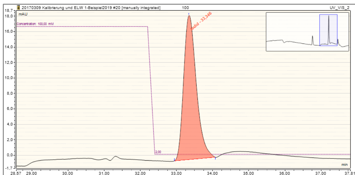
Abbildung 4-4. Beispiel eines Chromatogramms der Kalibrierung zur Bestimmung des Iodids mittels Ionenchromatographie (IC)
