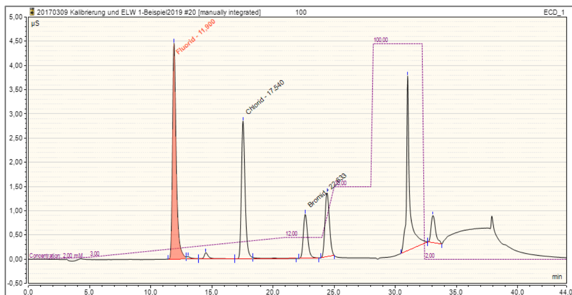
Abbildung 4-3. Beispiel eines Chromatogramms der Kalibrierung zur Bestimmung von Fluorid, Chlorid und Bromid mittels Ionenchromatographie (IC)
