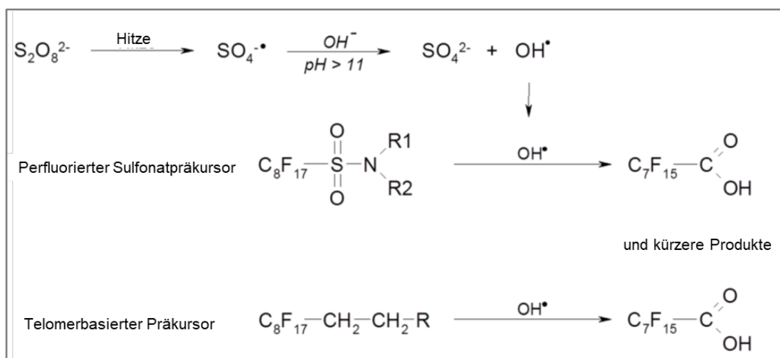
Abbildung 3-4. Schema der chemischen Oxidation der Präkursoren
