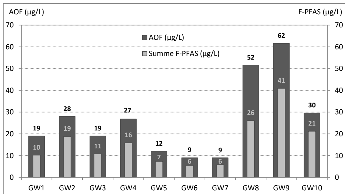
Abbildung 4-8. AOF- und F-PFAS-Werte in mit PFAS verunreinigtem Grundwasser
