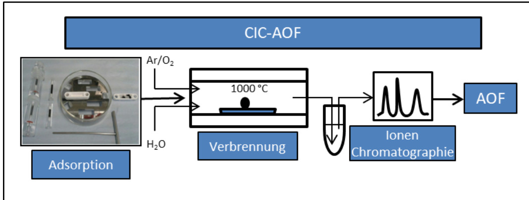
Abbildung 3-1. Schematische Darstellung der Verbrennungs-Ionen-Chromatographie (CIC) zur Bestimmung von adsorbierbarem organisch gebundenem Fluor (AOF) (von Abercron et. al., 2019)
