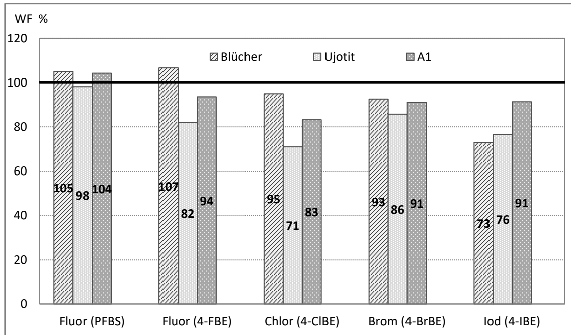
Abbildung 4-1. Einfluss der Aktivkohle (AK) auf die Wiederfindung (WF) von Standardsubstanzen
