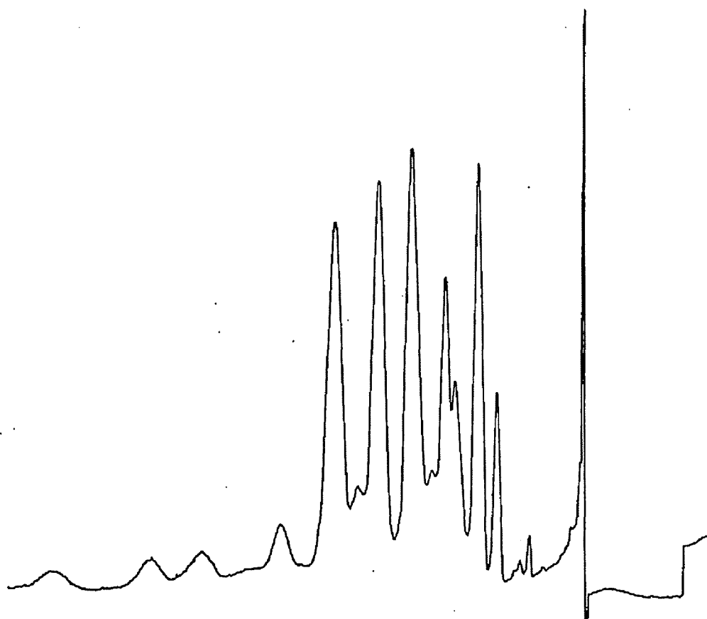
Fig 4 G.L.C.-E.C. Chromatogram Aroclor 1254
