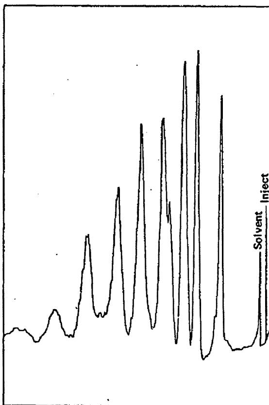
Fig 7 G.L.C.-M.C. Chromatogram Aroclor 1254
