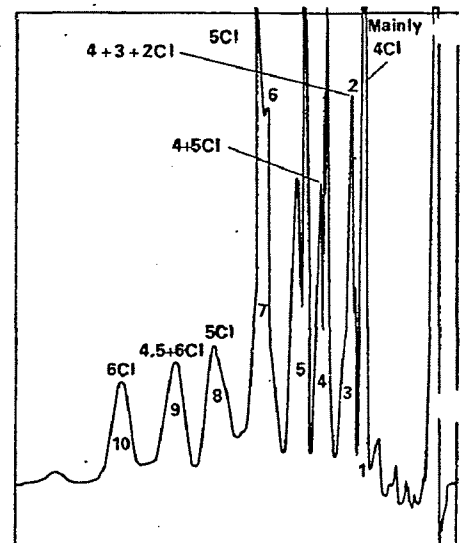
Fig 10 Aroclor 1254 F.I.D.-M.S. split
