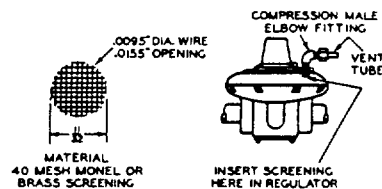
FIG. 11—Flame Check
