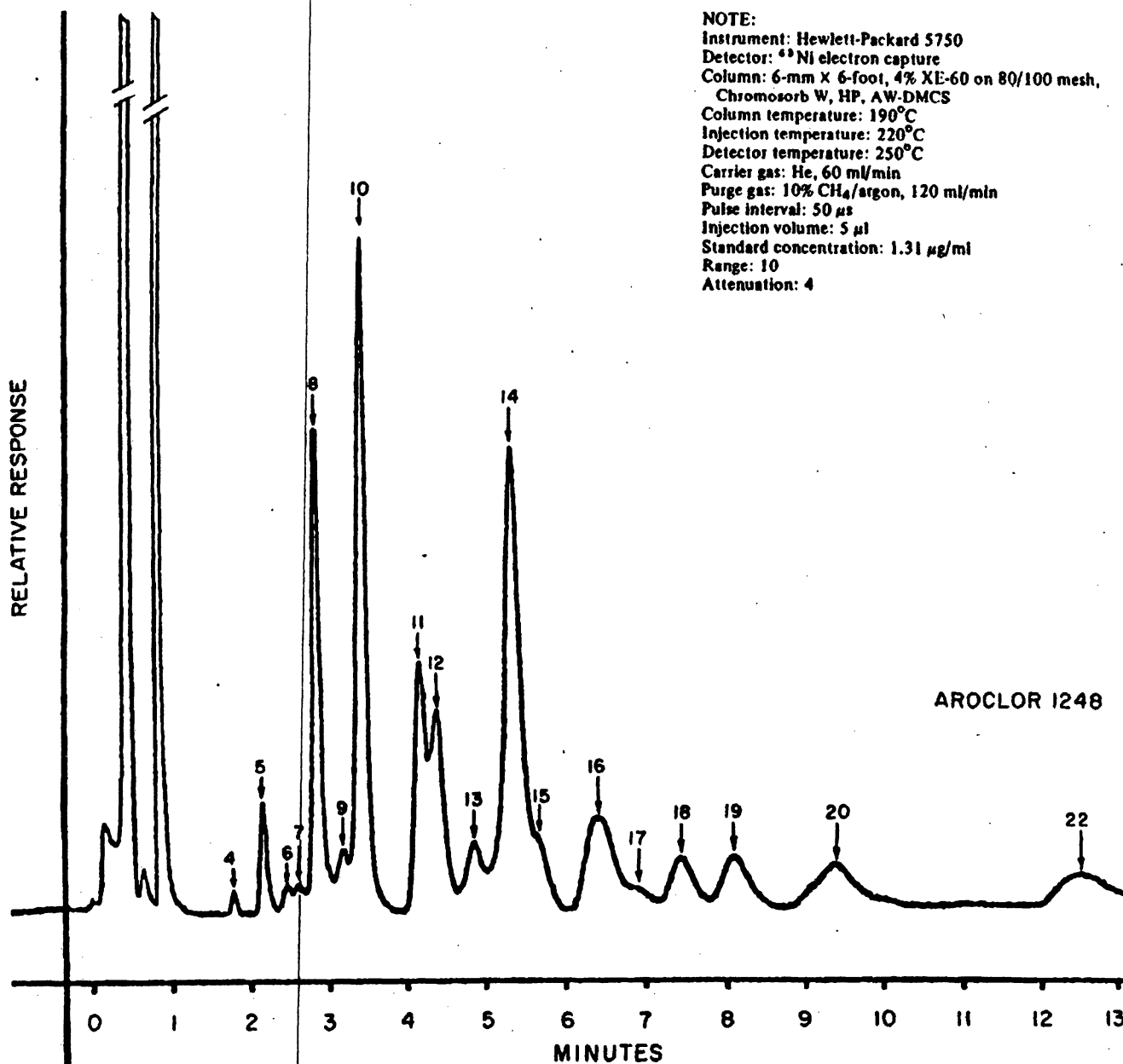
Fig. B5 Aroclor 1248 Electron Capture Chromatogram
