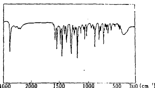
Fig. 4. IR Spectrum of \text{M-A}_2 (KBr)
