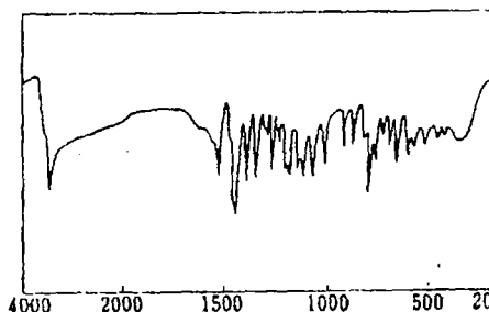
Fig. 3. IR Spectrum of \text{M-A}_1 (KBr)
