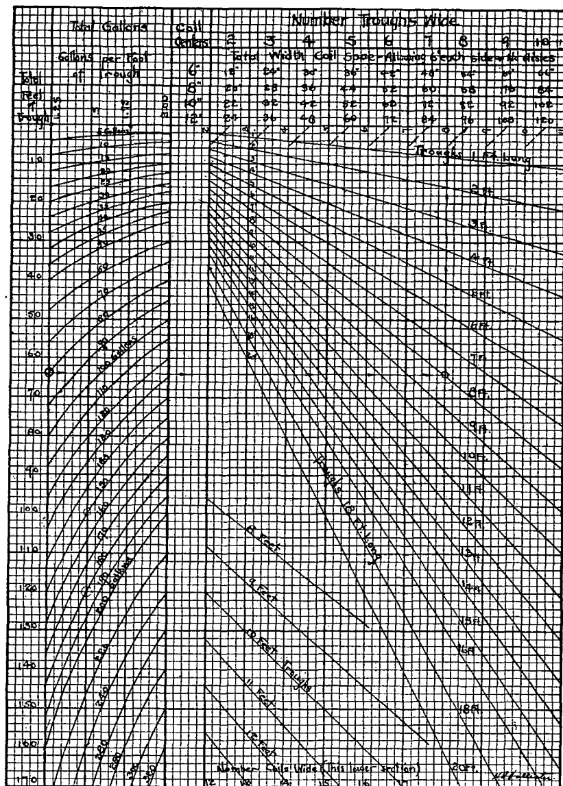
FIG. 80. TROUGHS
