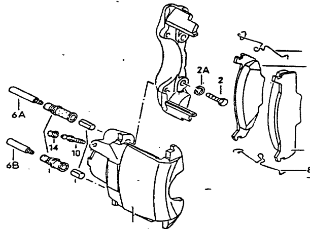
VW II sadel (Faustsattel)
