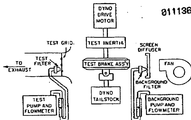
Fig. 1 - Dynamometer test schematic
