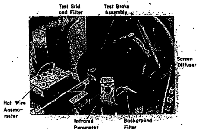
Fig. 2 - Dynamometer test setup
