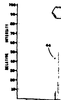
Figure 5. M. Aroclor 1232.
