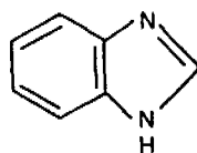
benzimidazole
