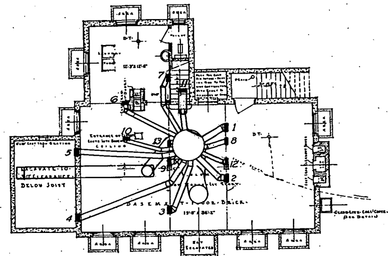
FIG. 56. BASEMENT PLAN
