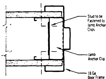
Door Details
