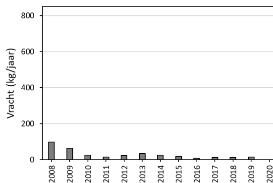
PFOS VROUWZD
