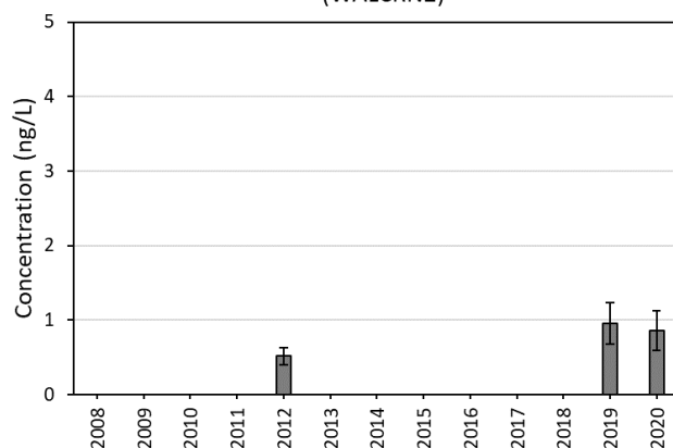
PFOS (WALCRN2)
