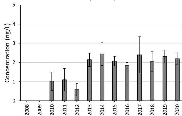
PFHpA (IJMDN1)
