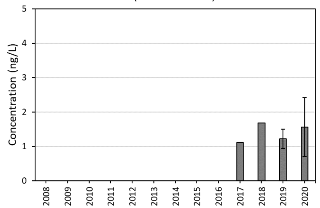
GenX (SCHAARVODDL)
