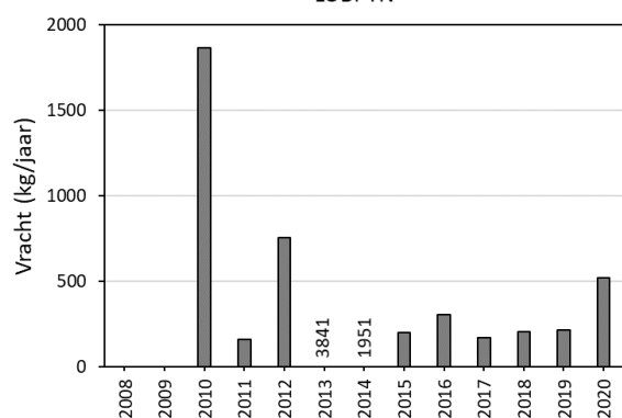
PFBA LOBPTN
