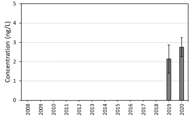
PFBA (WALCRN2)
