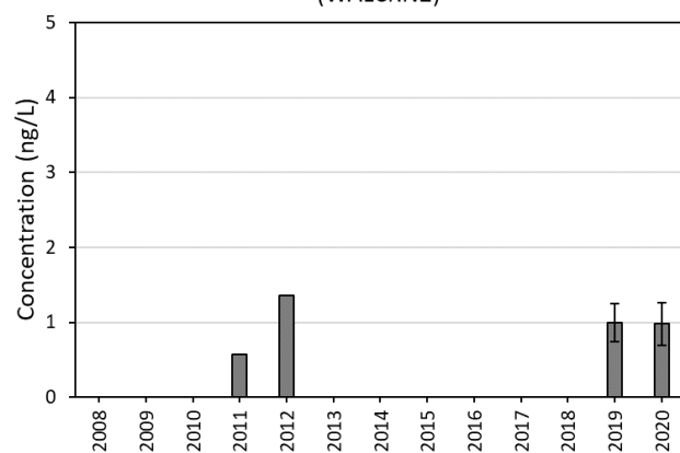
PFOA (WALCRN2)
