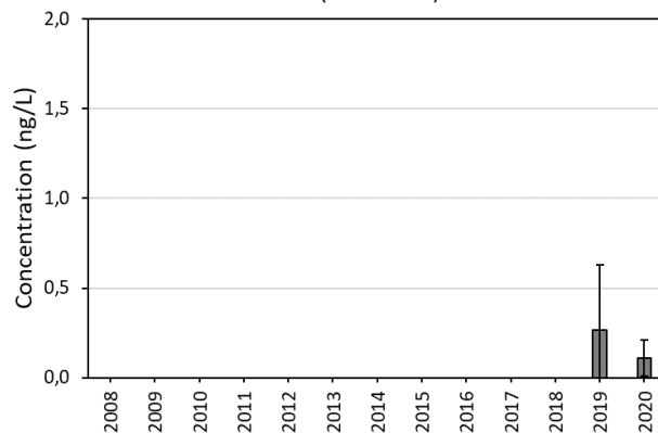
6:2 FTS (WALCRN2)
