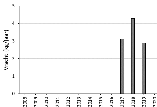
EtFOSAA IJMDN1
