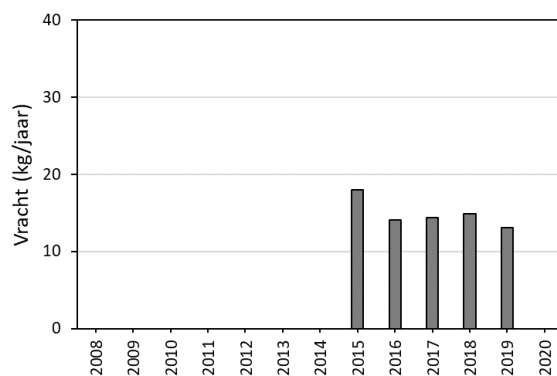
PFNA IJMDN1
