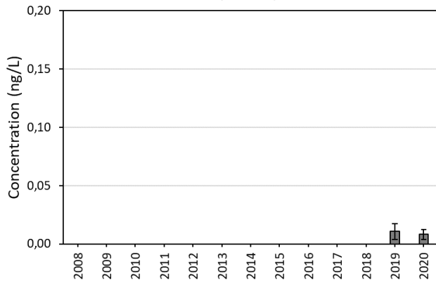
EtFOSAA (DREISR)
