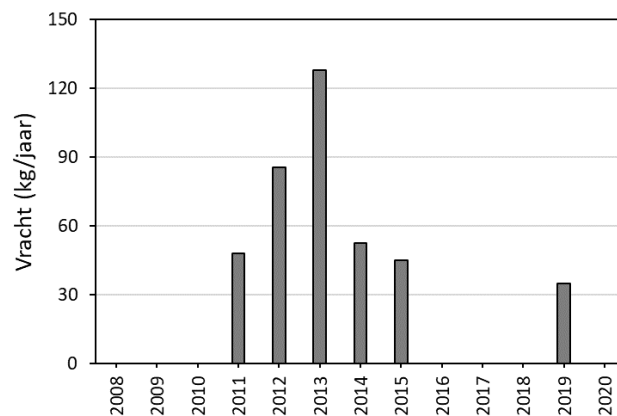
PFOA HARVSS
