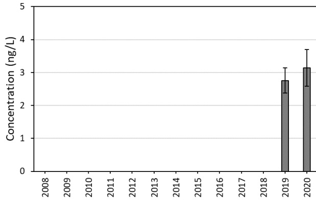
PFBA (DREISR)
