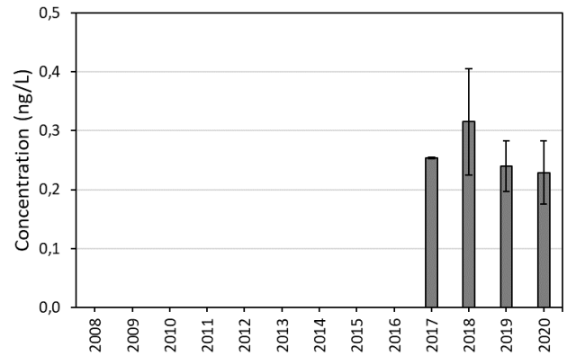
PFPeS (NIEUWGN)
