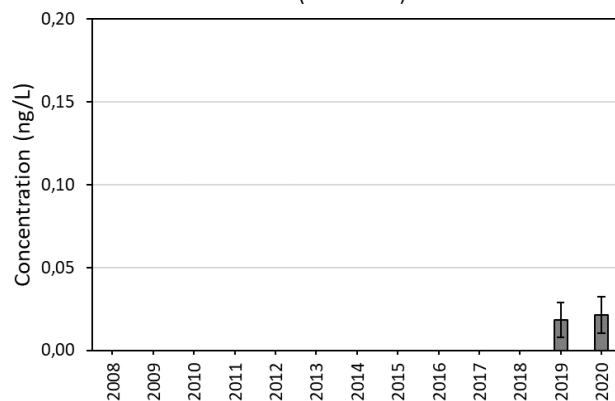
EtFOSAA (WALCRN2)
