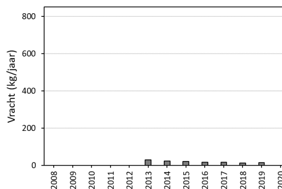
PFOS VROUWZD
