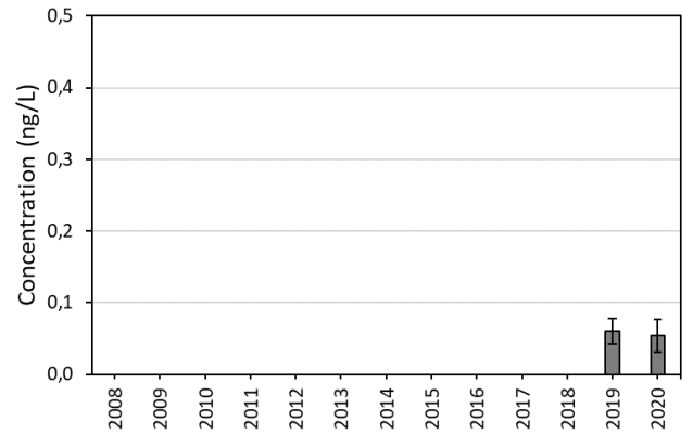
PFPeS (WALCRN2)
