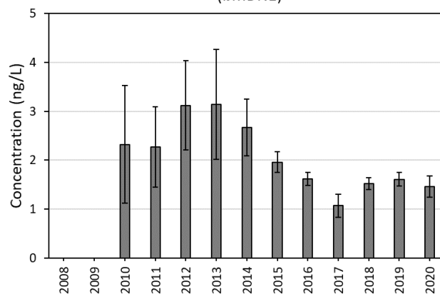
PFHxS (IJMDN1)
