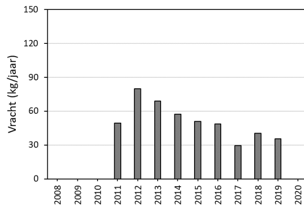
PFOA KEIZVR
