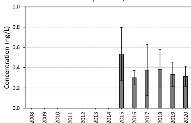
PFNA (EIJSDPTN)
