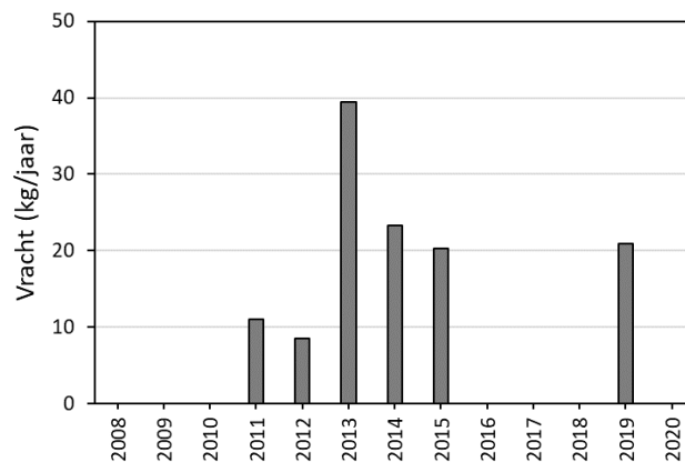
PFHpA HARVSS
