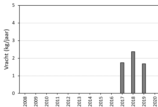
PFPeS KEIZVR
