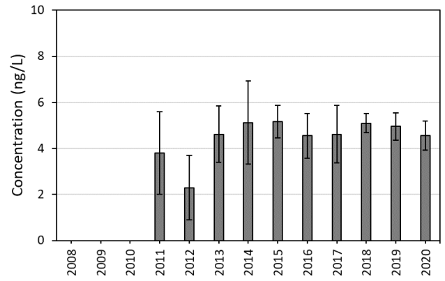
PFHpA (SCHAARVODDL)
