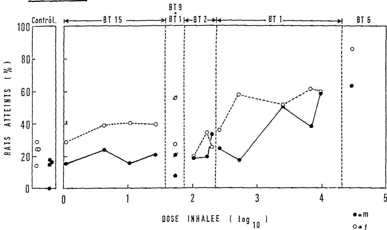
FIGURE 14 : proportion de rats atteints de cancer(s) en fonction de la dose
