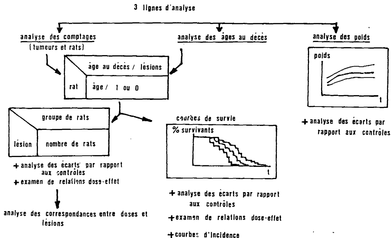
FIGURE 3 : plan de l'analyse statistique (analyse des données)
