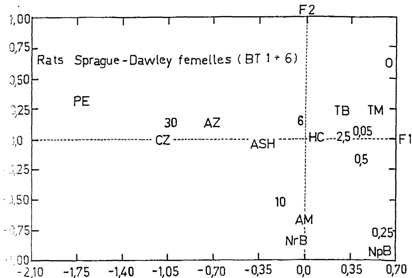
FIGURE 22 : analyse factorielle des correspondances entre les points-images des doses et les points-images des tumeurs. AZ = adénocarcinome mammaire ; ASH = angiosarcome du foie ; AZ = adénome de la glande de Zymbal ; CZ = carcinome de la glande de Zymbal ; HC = hépatocarcinome ; PE = papillome de l'estomac ; NpB = néphroblastome ; NrB = neuroblastome ; TB = tumeurs bénignes ; TM = tumeurs malignes. Les doses sont exprimées en 103 ppm, 4 h/j, 5 j/sem, pendant 1 an.
