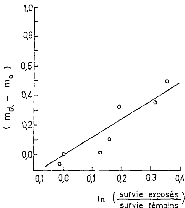
FIGURE 20 : corrélation entre la surmortalité et l'accroissement des tumeurs dues au VC ( r = -0,94 ). m_d est le nombre moyen de tumeurs par animal exposé à la dose d ; m_o est le nombre moyen de tumeurs chez les témoins. On a ajusté une droite passant par l'origine.
