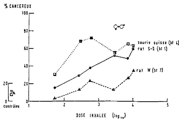
FIGURE 26 : comparaison interspèces dans les études du Pr MALTONI.
