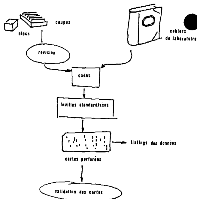
FIGURE 2 : plan de l'analyse statistique (collecte des données)
