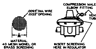
FIG. 11—Flame Check
