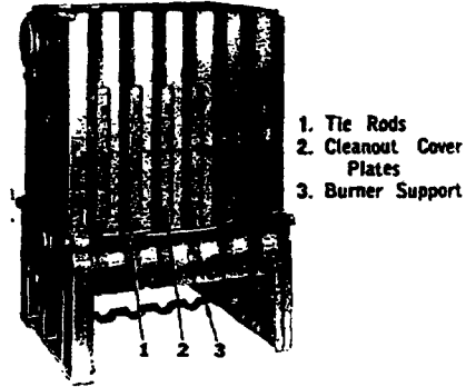
FIG. 3—Section Assemblage
