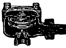
Fig. 6. Webster Size 782 Trap
