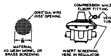
FIG. 11—Flame Check
