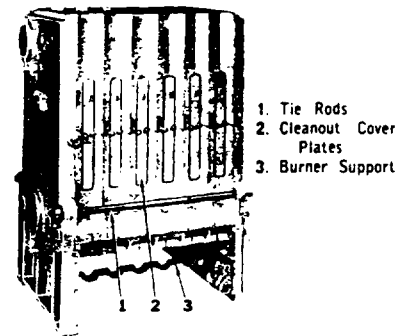
FIG. 3—Section Assemblage
