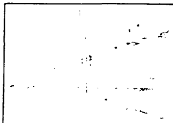
A. Chrysotile
