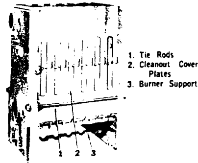
FIG. 3—Section Assemblage
