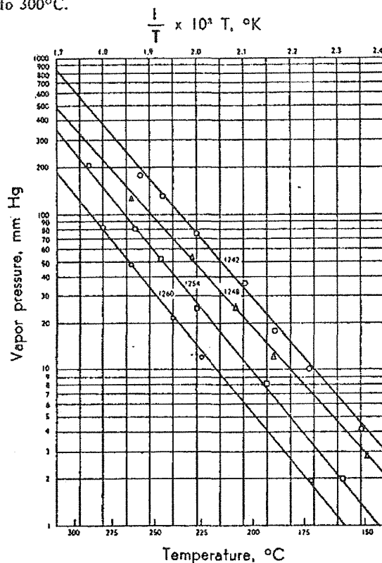
Fig. 3—VAPOR PRESSURES OF AROCLORS
