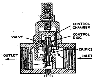
FIG. 30. IMPULSE TRAP
