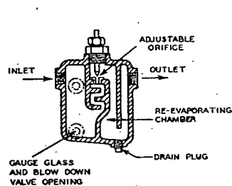
FIG. 29. FLASH TRAP
