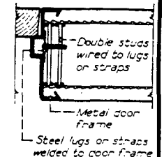
Jamb D
