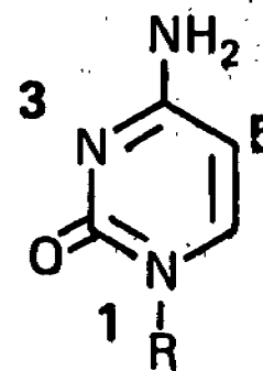
Cytosine
