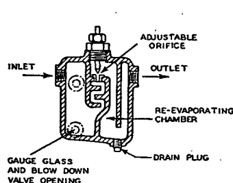
FIG. 29. FLASH TRAP
