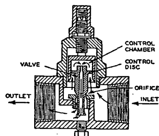
FIG. 30. IMPULSE TRAP
