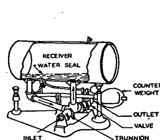
FIG. 31. TILTING TRAP
