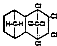
ALDRIN
