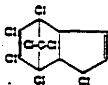
HEPTACHLOR
