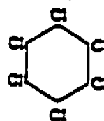
LINDANE
