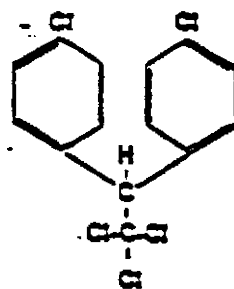
DDT
