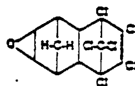
ENDRIN
